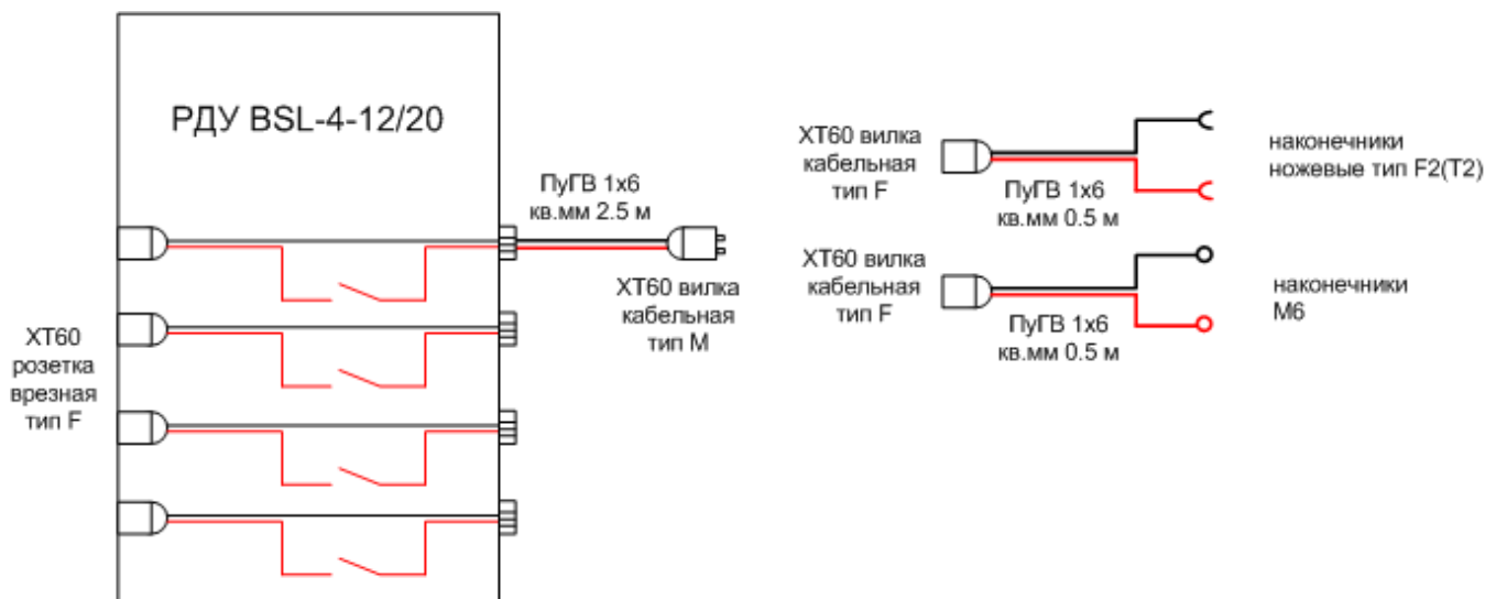
Рис 3.1 Комплект силовых кабелей РДУ CONBAT BSL-4-12/20
