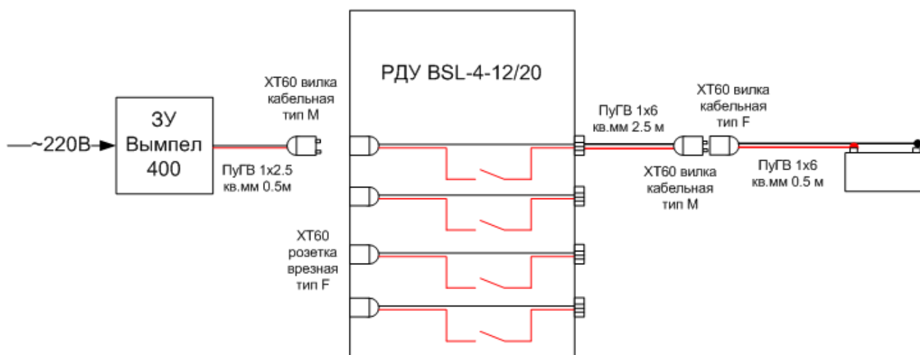
Рис 3.3 Схема подключения РДУ CONBAT BSL-4-12/20
