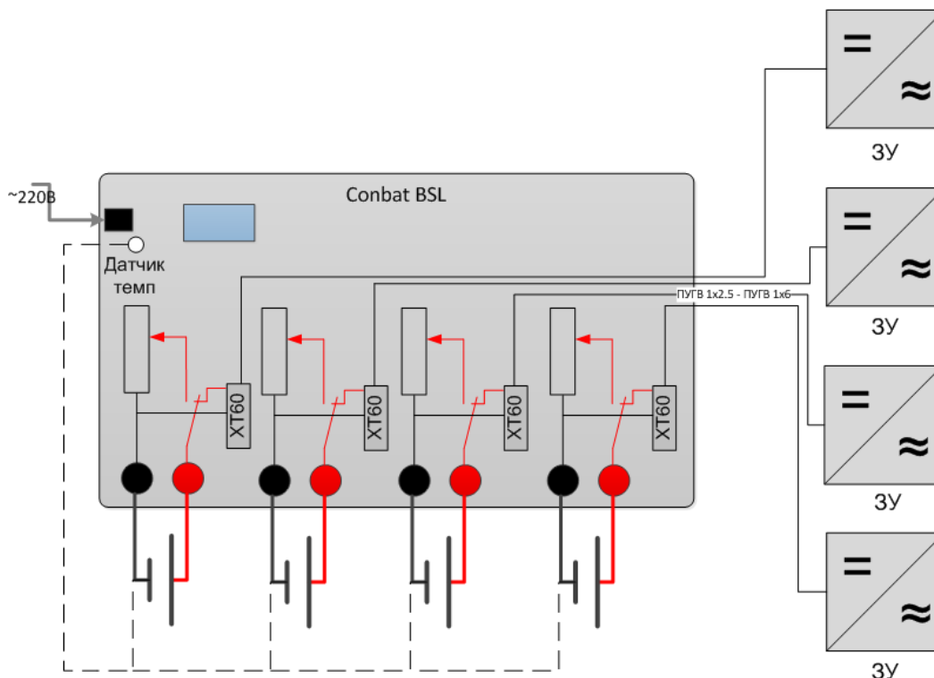
Рис 3.4 Принципиальная схема работы и схема подключения РДУ CONBAT BSL-4-12/20
