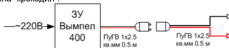
Рис 3.2 Комплект силовых кабелей ЗУ Вымпел-400
